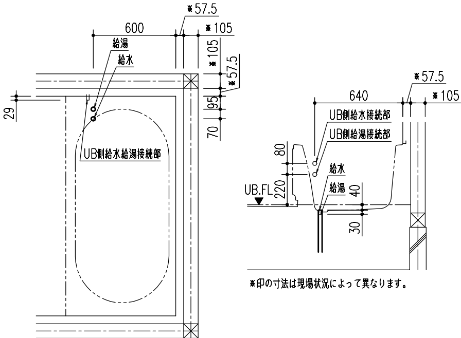
給水給湯配管立上げ位置 点検口止め
