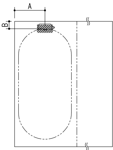
追いだき配管立上位置図
